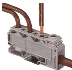
монтаж провода
